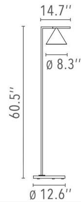
F1530059 Brass
